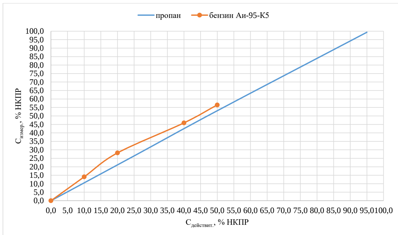
Рисунок А.3 - ИДК-10-Х1. Перекрестная чувствительность бензина АИ-95 к пропану
