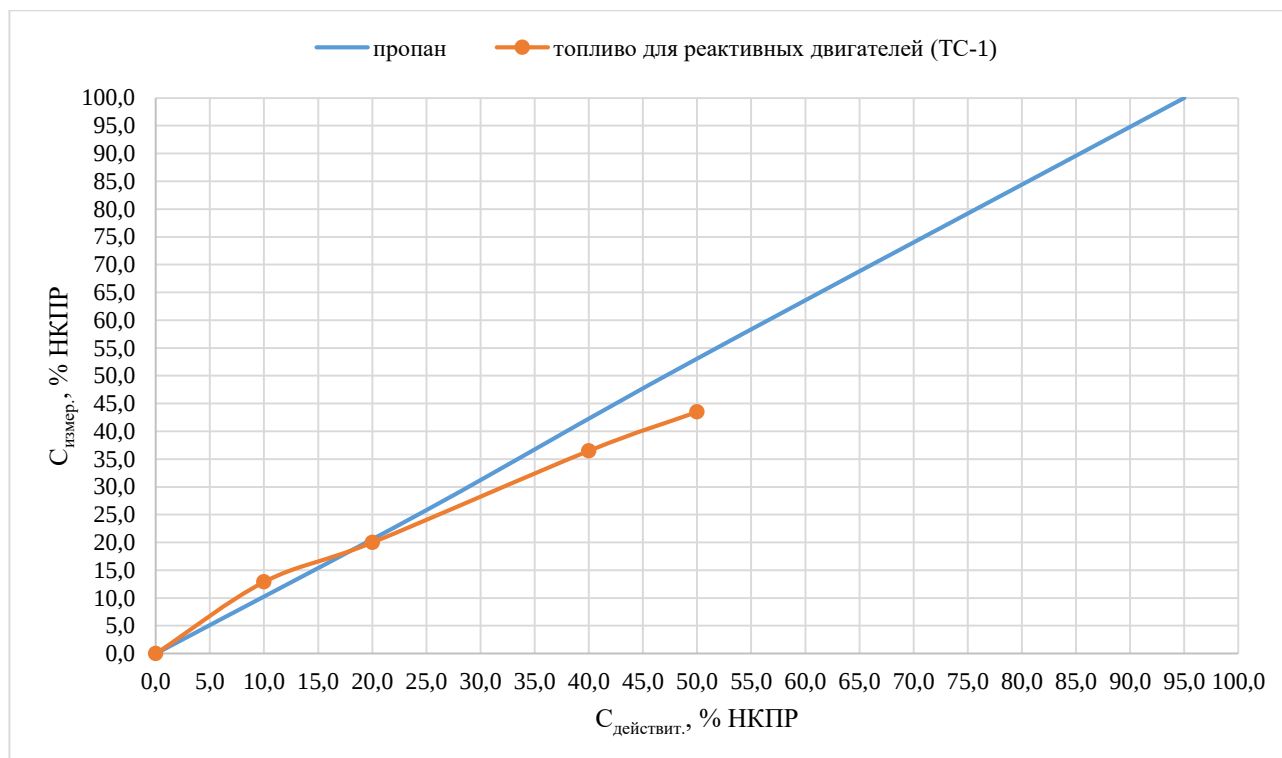
Рисунок А.5 - ИДК-10-X1. Перекрестная чувствительность керосина ТС-1 к пропану
