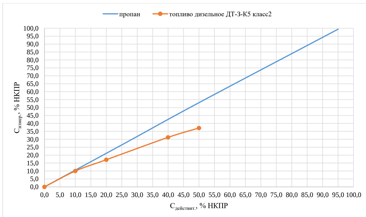
Рисунок А.4 - ИДК-10-Х1. Перекрестная чувствительность топлива дизельного к пропану
