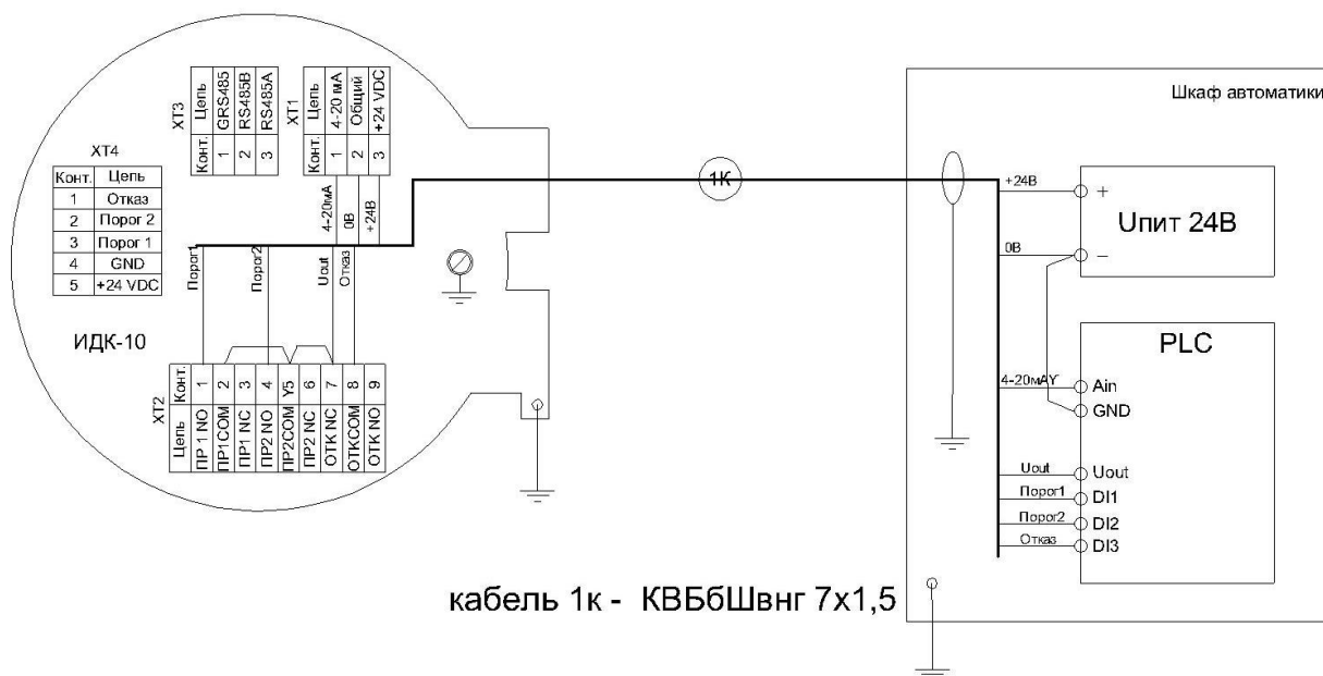
Рисунок Д.3 – Пример схемы внешних подключений ИДК-10 одним кабелем (только при коммутации дискретными выходами напряжение постоянного тока до 30 В)
