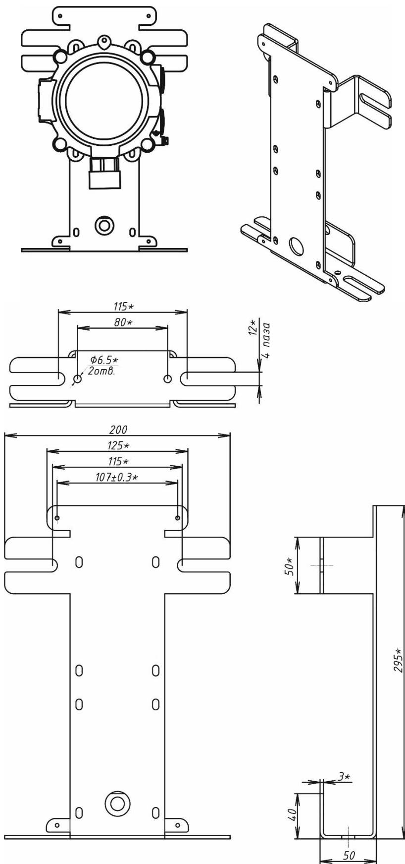
Рисунок Б.6 – Пластина монтажная ОФТ.18.2272.00.00.00 СИ68
