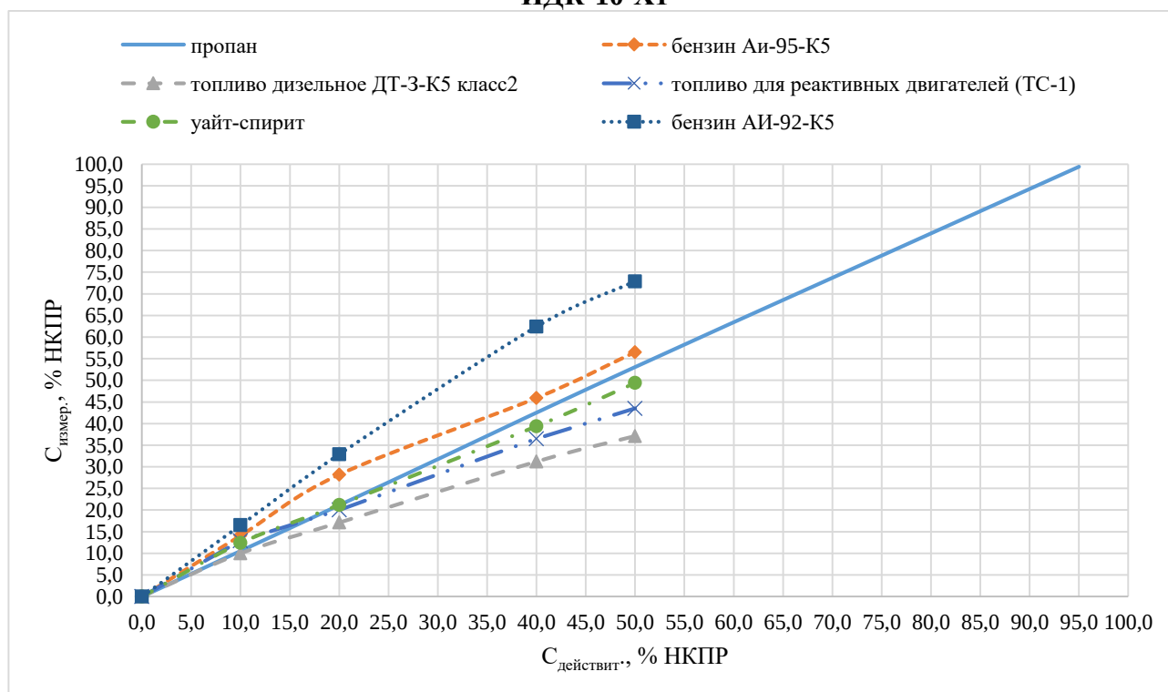
Рисунок А.1- ИДК-10-X1. Перекрестная чувствительность паров нефтепродуктов к пропану
