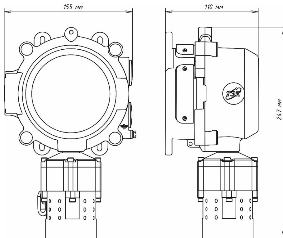
Рисунок Б.3 – ИДК-10-X3
