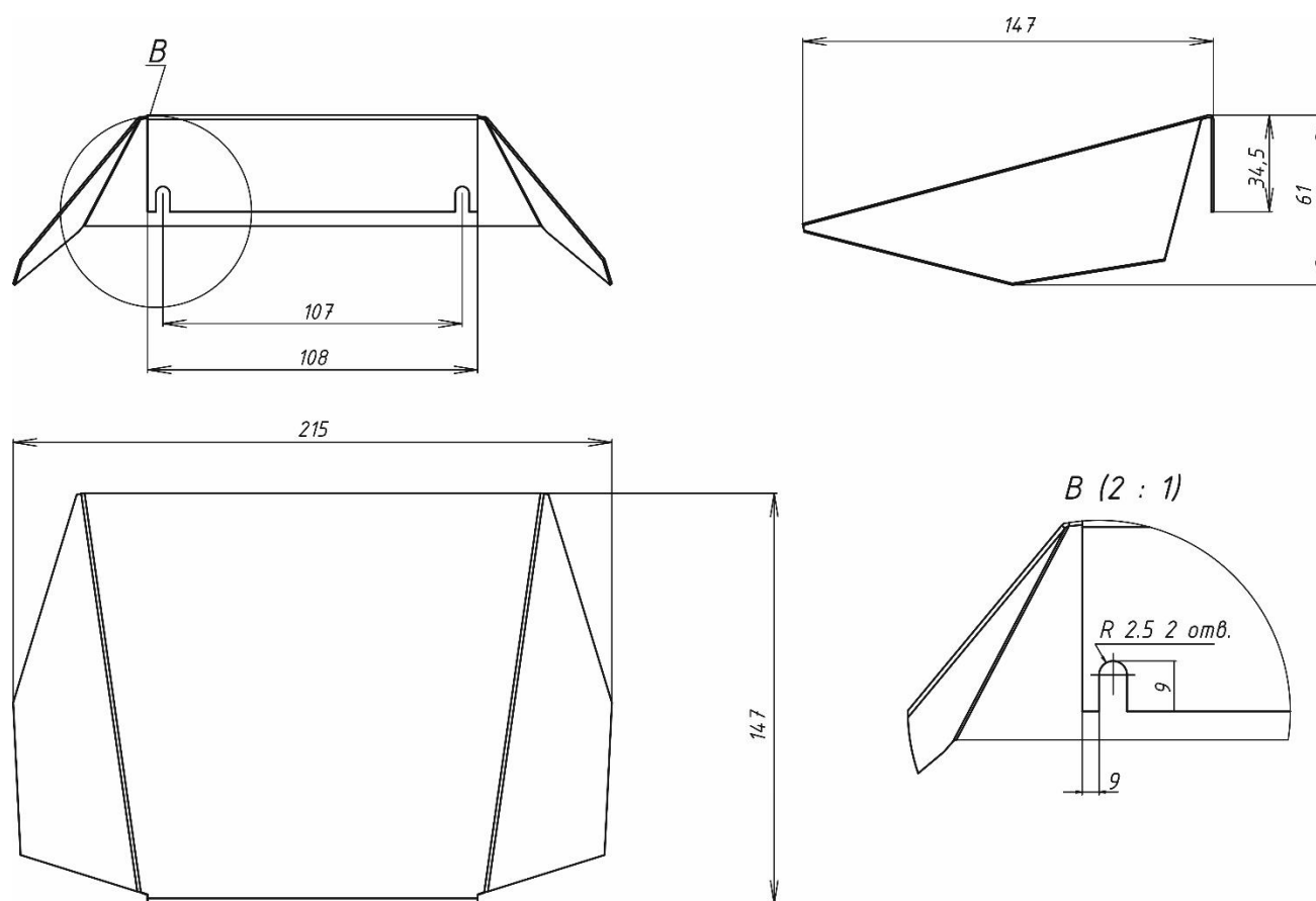
Рисунок Б.8 – Козырек ОФТ.18.2272.00.00.00 ЗИ57
