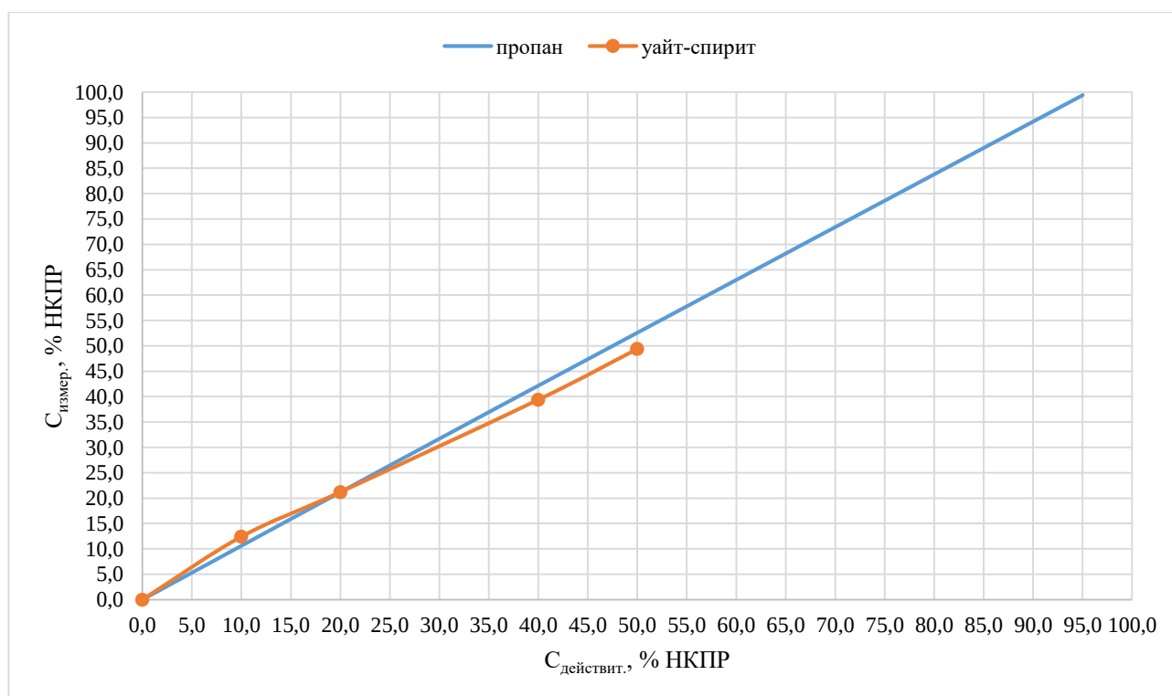
Рисунок А.6 - ИДК-10-X1. Перекрестная чувствительность уайт-спирита к пропану
