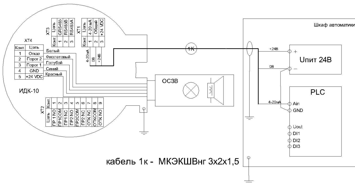
Рисунок Д.1 – Пример схемы внешних подключений ИДК-10
