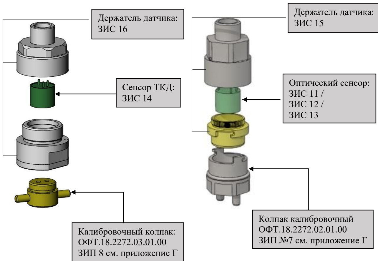
Рисунок И.2 – Блок сенсора
