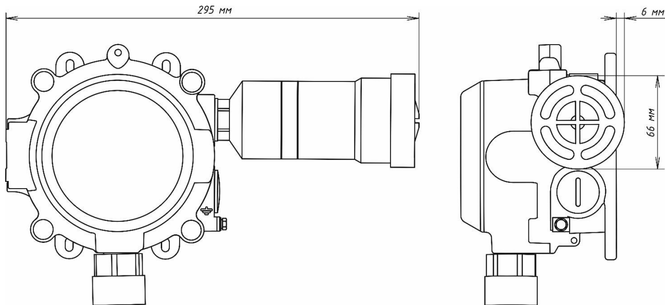
Рисунок Б.4 – ИДК-10-X1 с ОСЗВ
