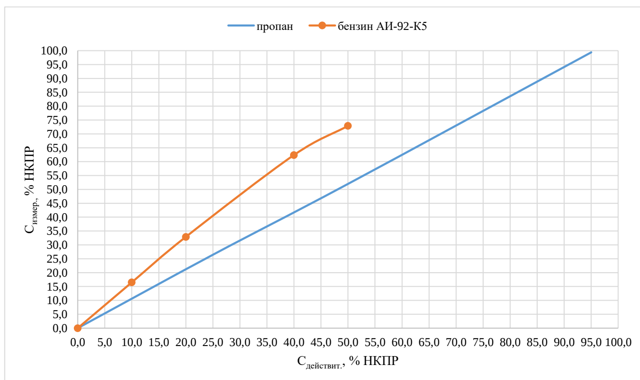
Рисунок А.2 - ИДК-10-X1. Перекрестная чувствительность бензина АИ-92 к пропану
